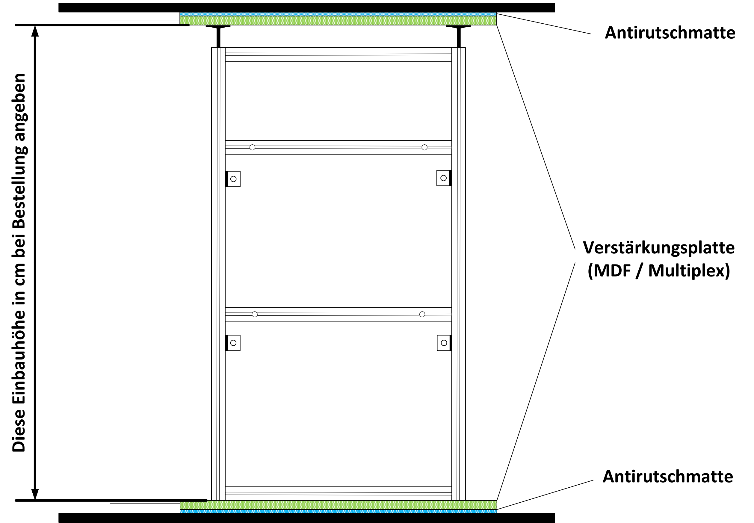
Beispiel: Einbau mit Verstärkung und Antirutschmatte
